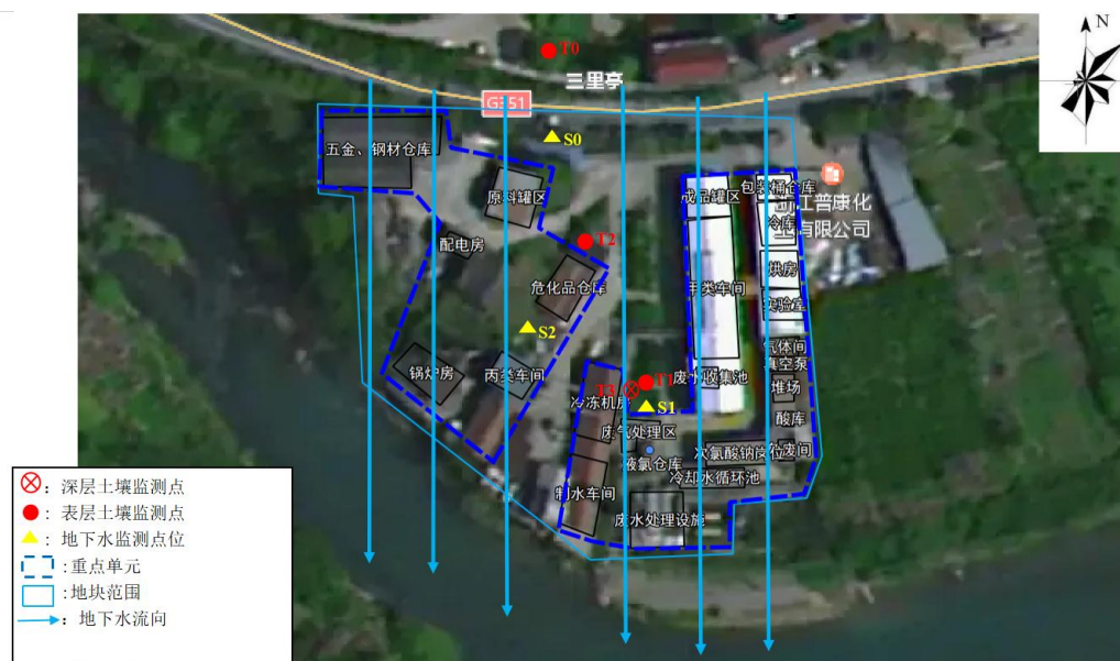
图 2.3-1 2024 年度土壤环境自行监测点位布设位置示意图
