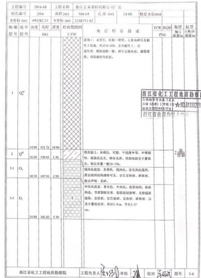
钻孔柱状图
