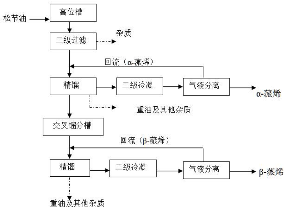
图 4.1-5 松节油精馏工艺及产污环节流程图
