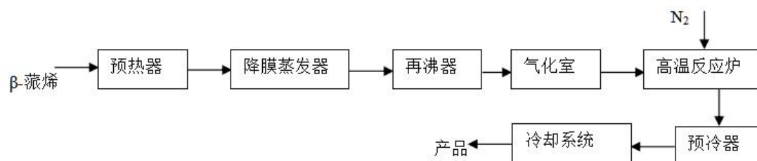
图 4.1-6 月桂烯生产工艺及产污环节图
