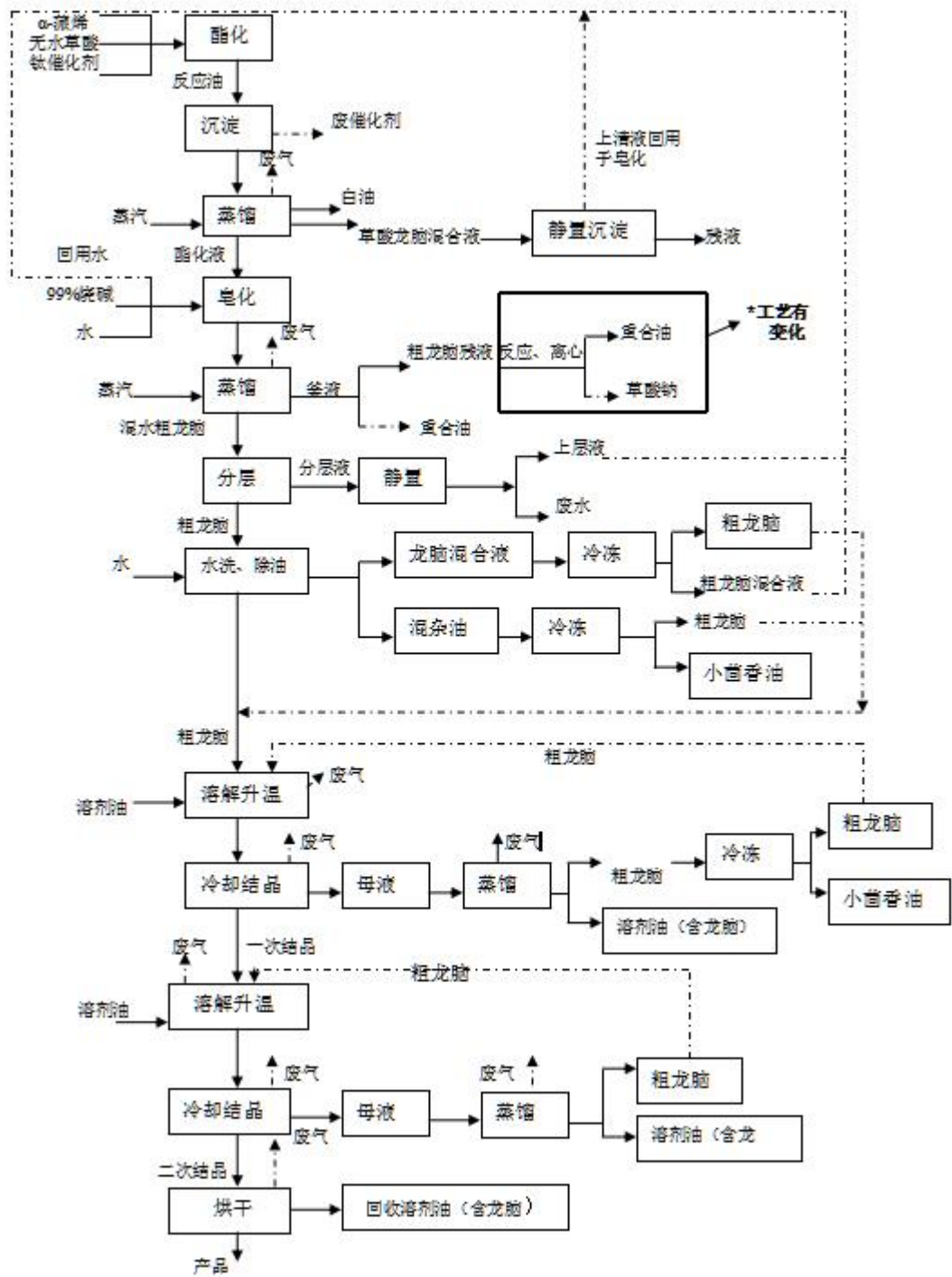
图 4.1-7 常规冰片生产工艺及产污环节图
