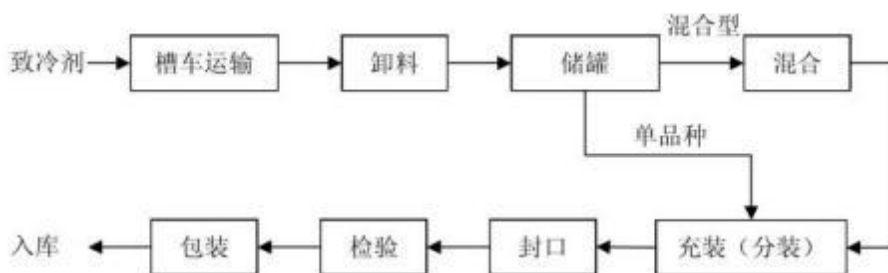
图 4.1-4 致冷剂分装工艺流程图
