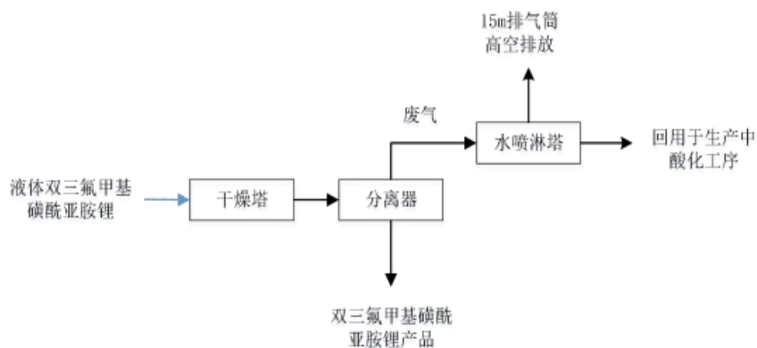
图 4.1-7 双三氟甲基磺酰亚胺锂盐干燥包装工艺流程及产污环节图
