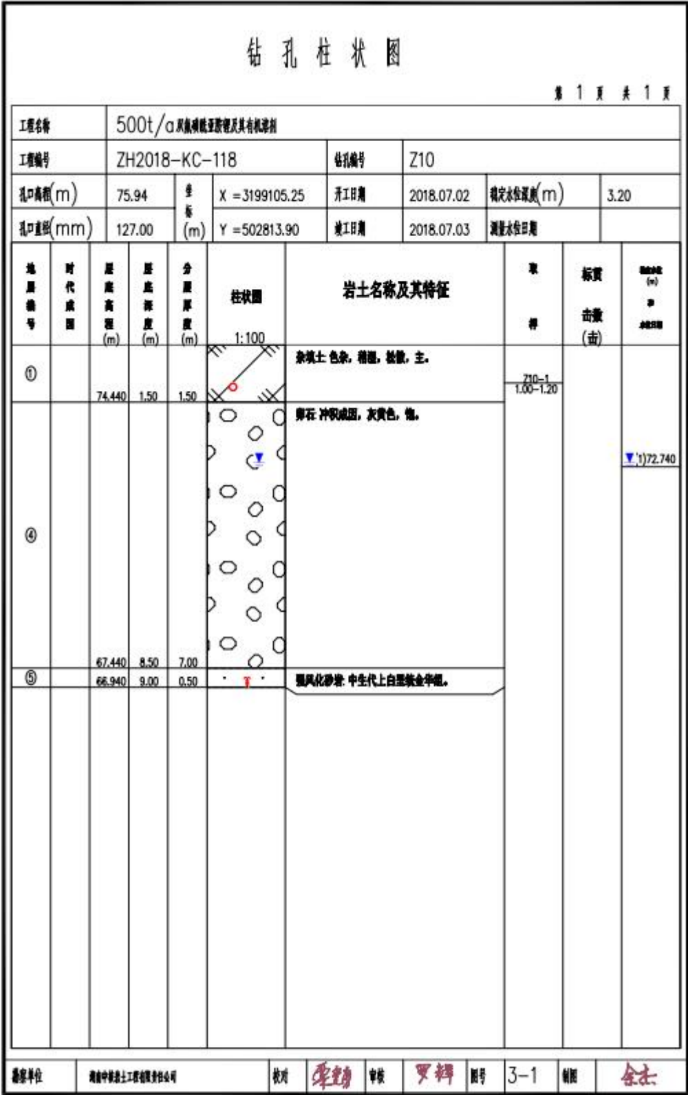
图 3.1-2 钻孔柱状图
